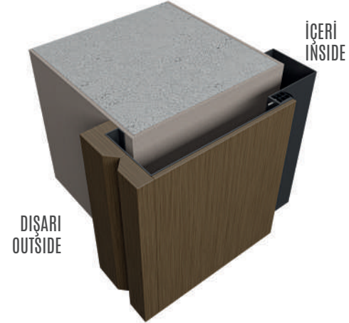
Fitel Altından Vidalamalı Kaplamalı Sabit Kasa HIDDEN SCREWED FIXED COVERED FRAME
